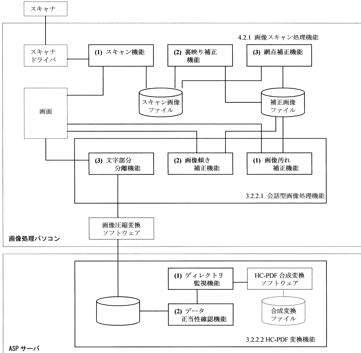
図2 システムブロック図
